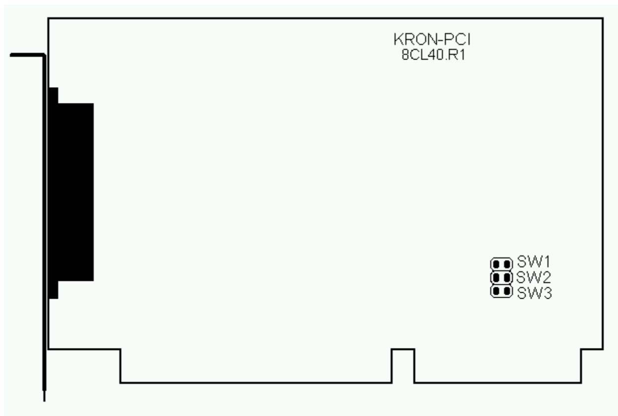
Рис.1. Переключатели адаптеров "4CL40 PCI ES16.R1", "4CL40 PCI ES128.R1", "8CL40 PCI ES16.R1", "8CL40 PCI ES128.R1".
